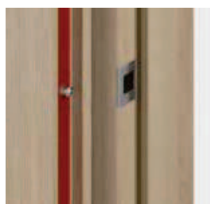
4 bolce antywyważeniowe uszczelka ogniowa (Typ II)
