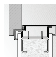
ościeżnica kąтова duża montaż na ścianie kartonowo-gipsowej
