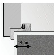
ościeżnica kąтова mała
