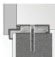
ościeżnica kąтова duża montaż na dyble
