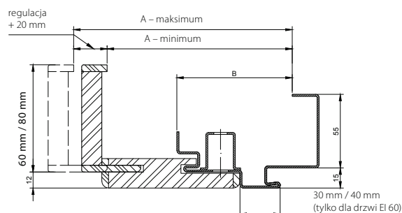
przekrój ościeżnicy PROJEKT
