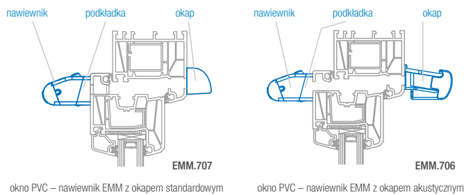
okno PVC – nawiewnik EMM z okapem standardowym
