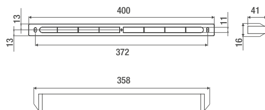
Mufa montażowa MTM (widok od wewnętrznej strony okna) - L5
