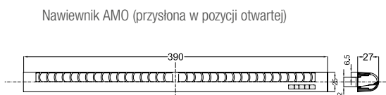
Nawiewnik AMO (przysłona w pozycji otwartej)
