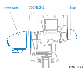
okno PVC – nawiewnik EXR z podkładką i okapem standardowym
