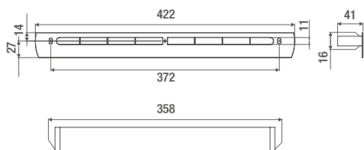
Mufa montażowa MTX (widok od wewnętrznej strony okna) - L4
