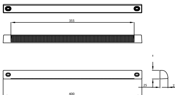
Okap standardowy AERECO
