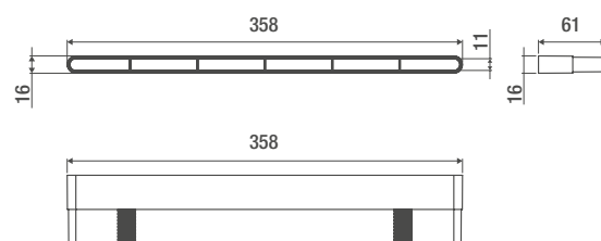
Przedłużenie do mufy montażowej MTX i MTM (element wewnątrz profilu okna) - L7
