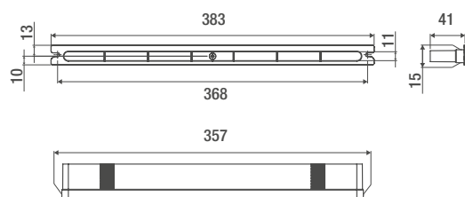
Mufa montażowa MTX i MTM (widok od zewnętrznej strony okna) - L6
