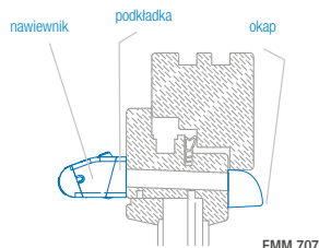
okno drewniane – nawiewnik EMM z okapem standardowym
